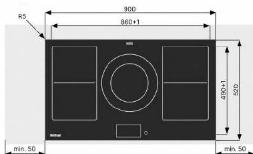
Aufliegender Einbau
