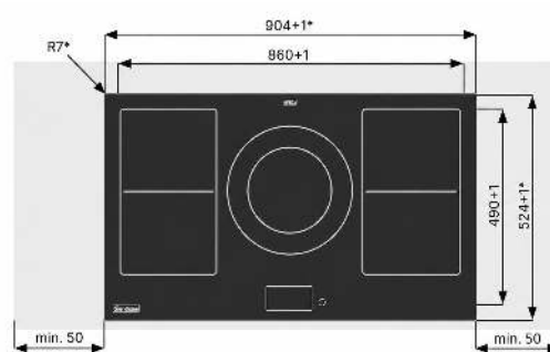
Flächenbündiger Einbau
