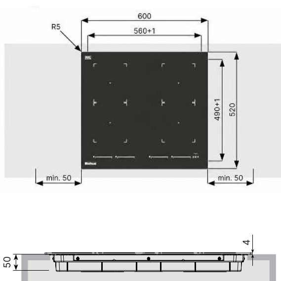
Aufliegender Einbau
