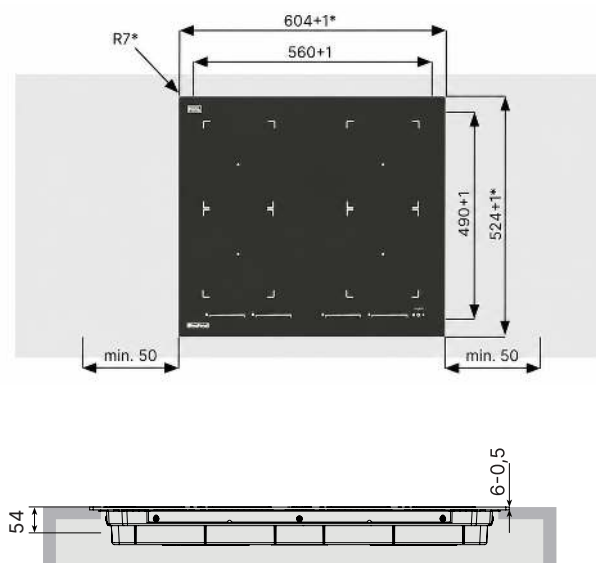
Flächenbündiger Einbau
