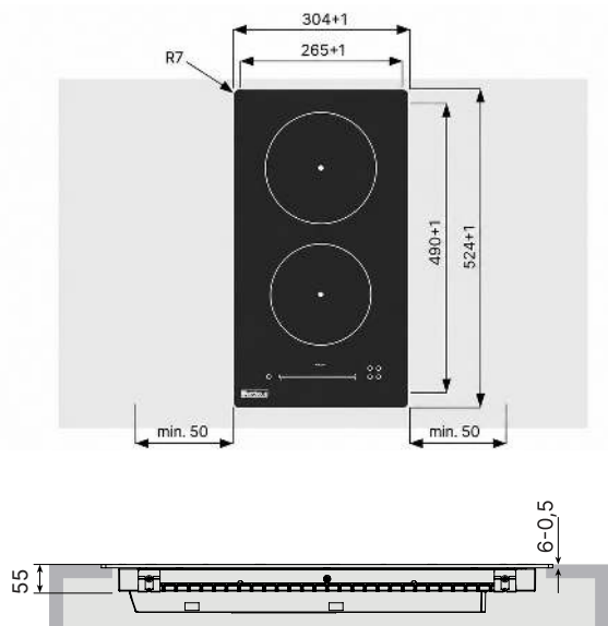
Flächenbündiger Einbau
