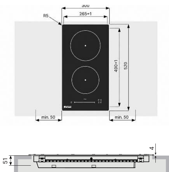
Aufliegender Einbau
