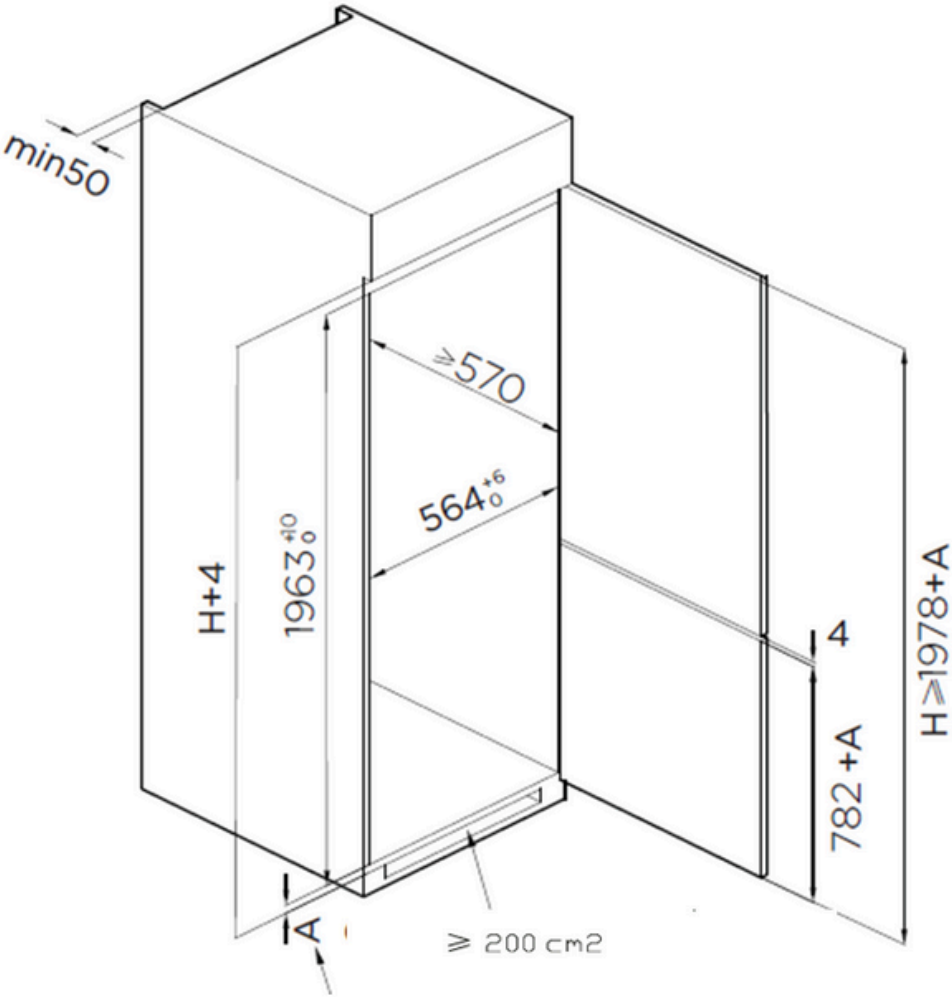
A- SHELF THICKNESS A- ÉPAISSEUR DE LA TABLETTE
